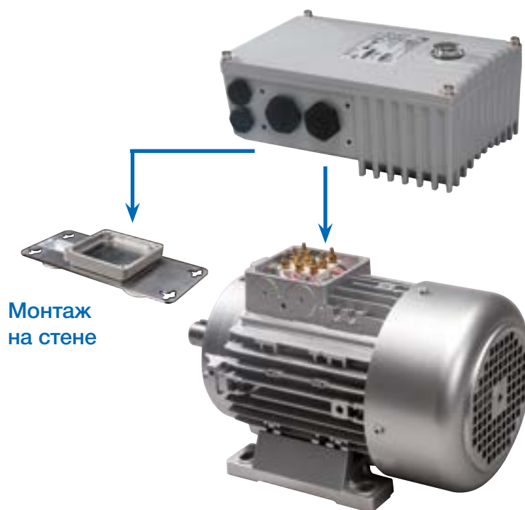
Монтаж на двигателе
