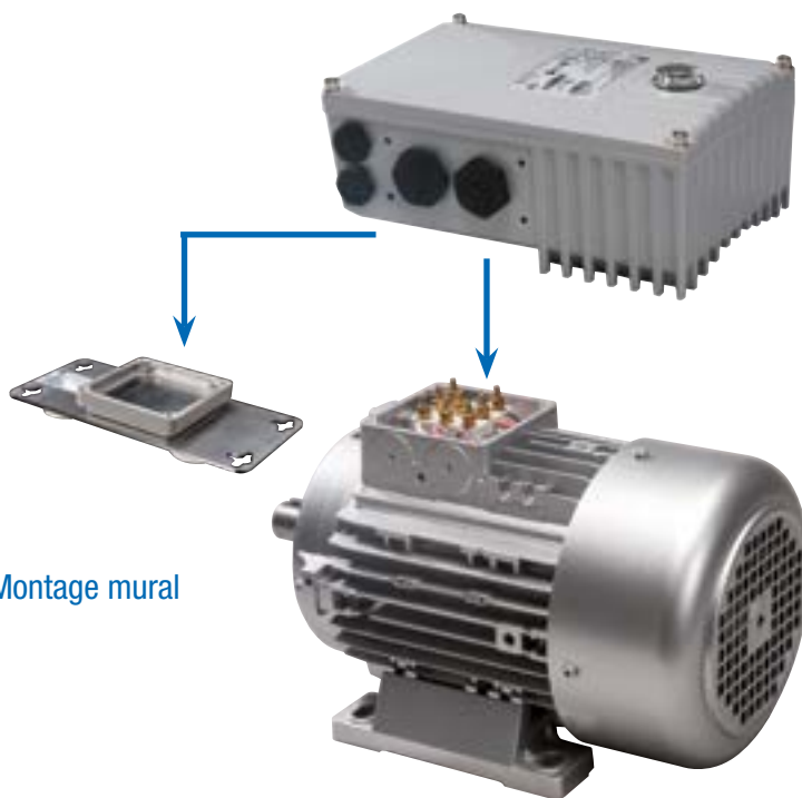
Montage moteur
