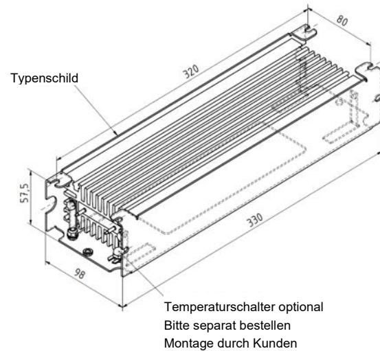
SK BR4-... Baugröße 4
