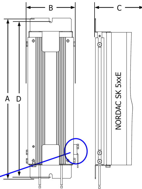
SK BR4-... Baugröße 2
