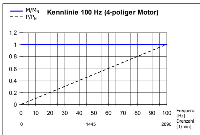
Abbildung 22: Kennlinie 100 Hz
