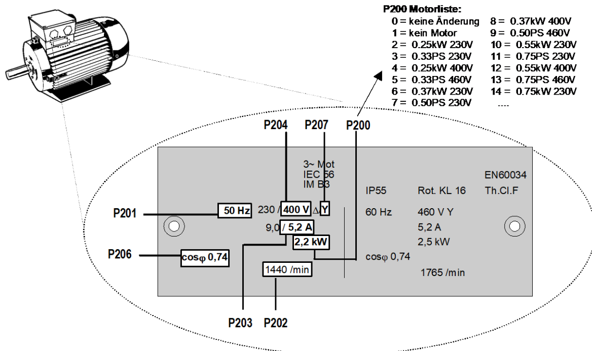
Abbildung 12: Motortypenschild
