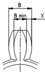
Kuva 29: ROTEX-sakarakytkimen hammaspaksuuden mittaaminen®
