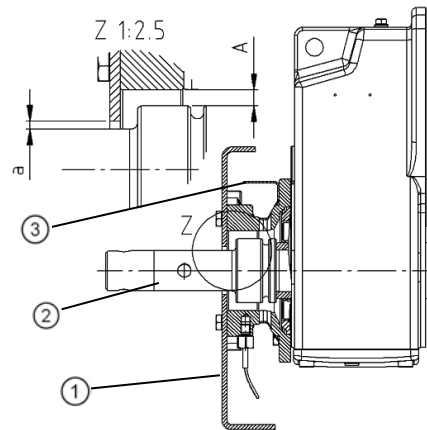
Kuva 13: SCX-laipan asennusesimerkki
