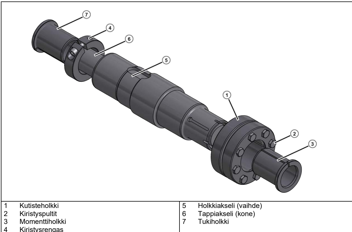
Kuva 12: GRIPMAXX™:n räjäytyskuva
