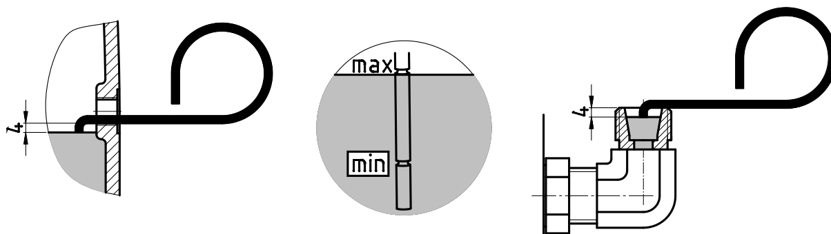
Kuva 27: Öljytason tarkistus öljytikulla
