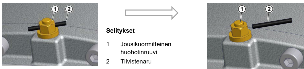
Kuva 21: Jousikuormitteisen huohotinruuvin aktivointi
