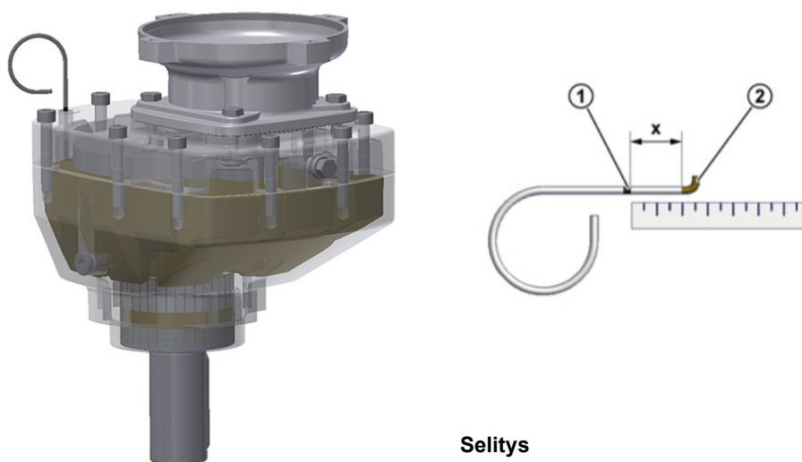
Kuva 36: Öljytaso SK 771.1 ... 1071.1
