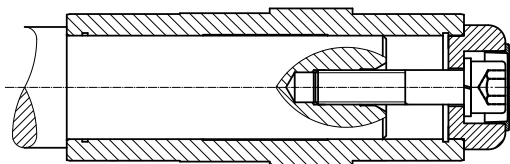
Kuva 6: Olakkeelliselle akselille kiinnityselementillä kiinnitetty vaihde
