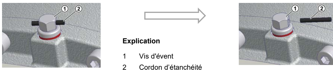
Figure 20: Activation de la vis d'évent
