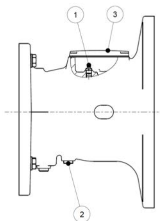
Figure 27: Regraissage de l'adaptateur IEC/NEMA AI et AN option BRG1
