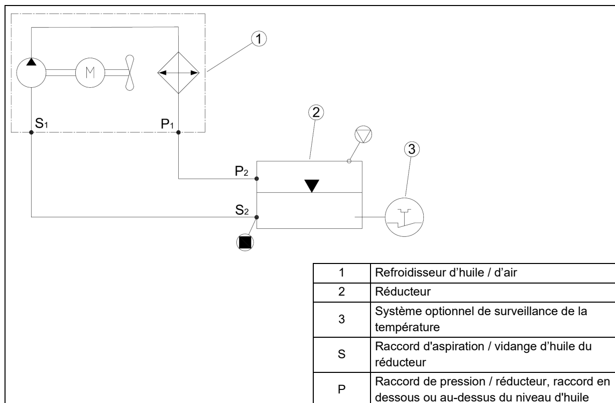
Figure 17: Connexion du refroidisseur d'huile / d'air
